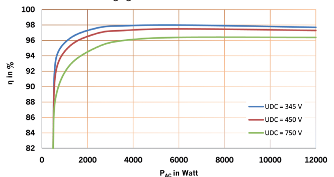
Wirkungsgradverlauf SOLPLUS 120
